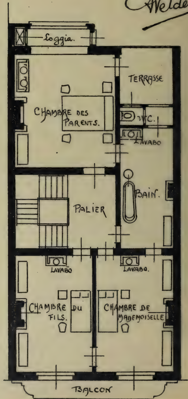
BEL ÉTAGE
